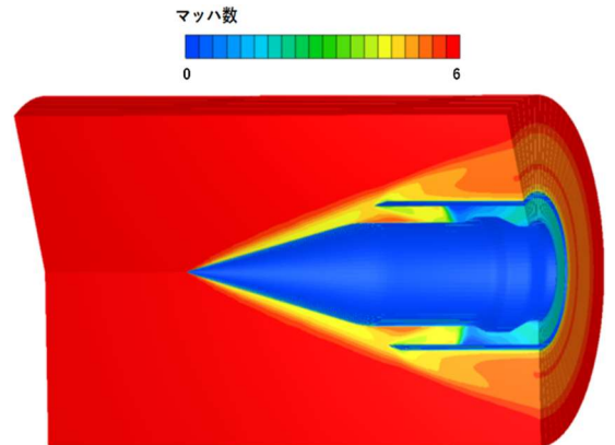
インテークの流れ計算結果
